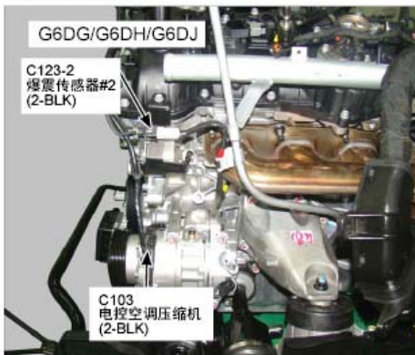
44. 发动机前左
