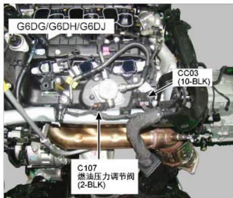
46. 发动机左侧
